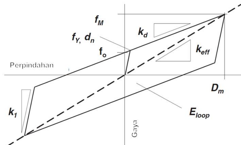
Gambar 14 – Properti nominal untuk isolator model gaya-perpindahan bilinear
